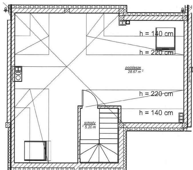
STRYCH
