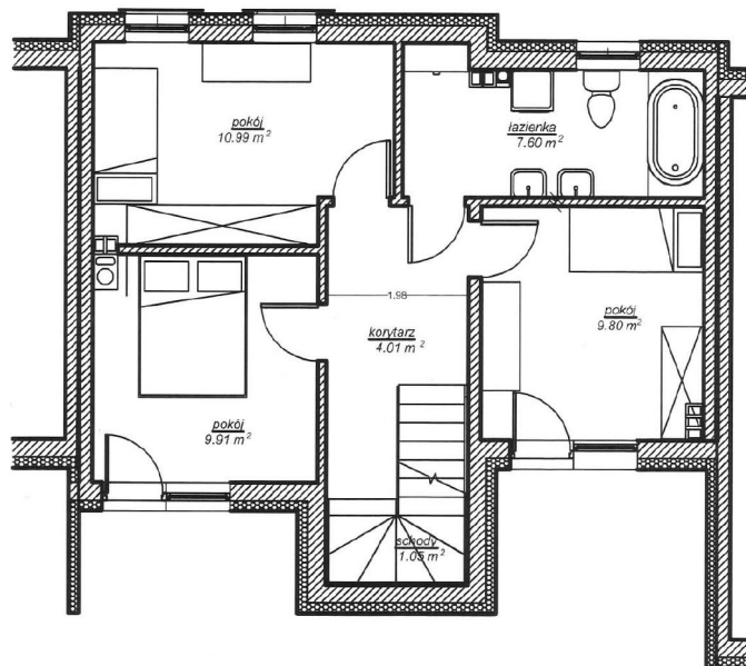
I PIĘTRO
